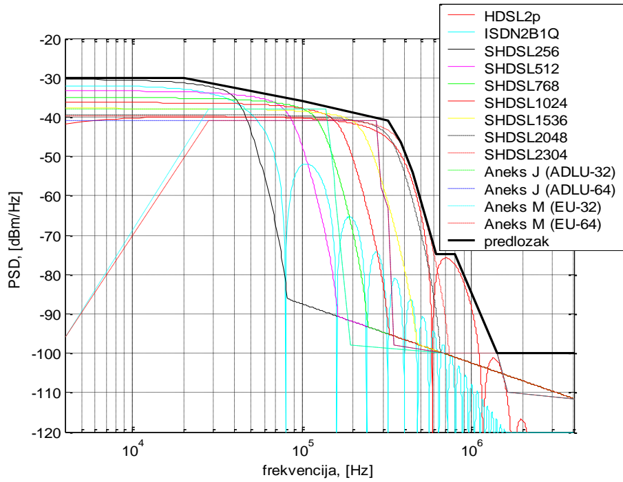
Slika 5.6.1 Frekvencijski predložak za odlazni smjer prijenosa (kratke pretplatničke linije).
