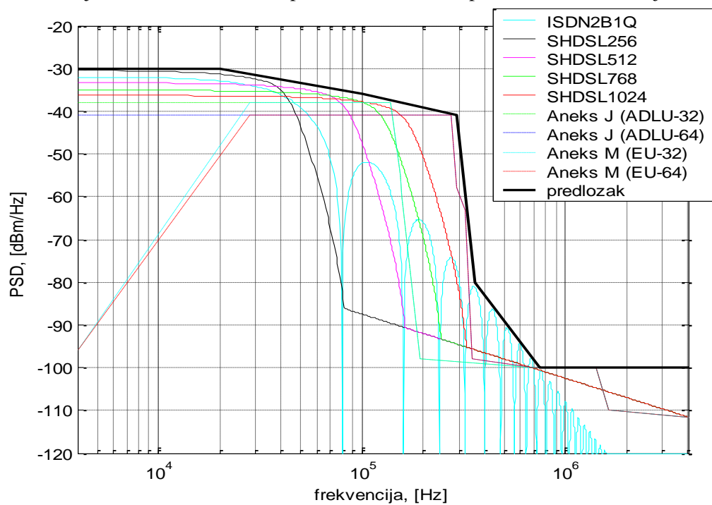
Slika 5.6.4 Frekvencijski predložak za odlazni smjer prijennosa (duge pretplatničke linije) za ADSL preko ISDN (aneks B).
