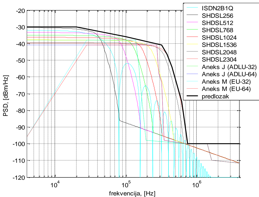
Slika 5.6.3 Frekvencijski predložak za odlazni smjer prijenosa (pretplatničke linije srednje duljine).
